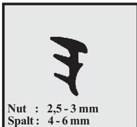
Profil-Nr. SD 2471 Farbe schwarz Material EPDM
