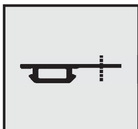
Profil-Nr. SD 2340 Farbe schwarz Material EPDM
