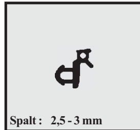
Profil-Nr. SD 2196 Farbe schwarz Material Silicon
