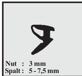
Profil-Nr. SD 2399 Farbe schwarz Material EPDM
