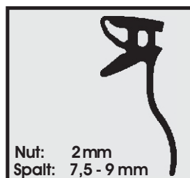
Profil-Nr. SD 2284 Farbe schwarz Material EPDM
