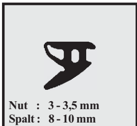
Profil-Nr. SD 2371 Farbe schwarz Material EPDM
