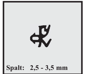
Profil-Nr. SD 2111 Farbe schwarz Material EPDM
