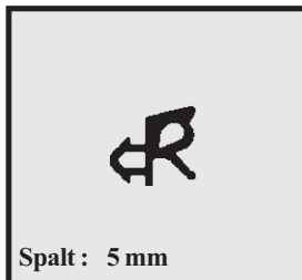
Profil-Nr. SD 2154 Farbe schwarz Material EPDM
