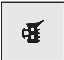
Profil-Nr. SD 2249 Farbe schwarz Material EPDM
