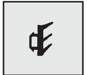
Profil-Nr. SD 2237 Farbe schwarz Material EPDM
