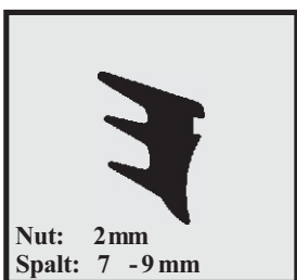
Profil-Nr. SD 2038 Farbe schwarz Material EPDM
