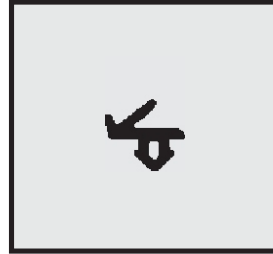
Profil-Nr. SD 2105 Farbe schwarz Material EPDM
