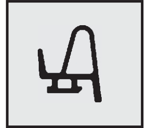
Profil-Nr. SD 2271 Farbe schwarz Material EPDM
