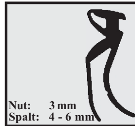
Profil-Nr. SD 2095 Farbe schwarz Material EPDM
