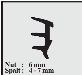
Profil-Nr. SD 2209 Farbe schwarz Material EPDM
