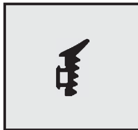
Profil-Nr. SD 2035 Farbe schwarz Material EPDM
