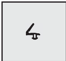
Profil-Nr. SD 2092 Farbe schwarz Material EPDM
