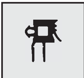
Profil-Nr. SD 2388 Farbe schwarz Material EPDM
