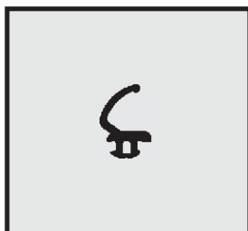
Profil-Nr. SD 2397 Farbe schwarz Material EPDM
