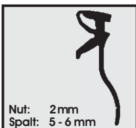
Profil-Nr. SD 2283 Farbe schwarz Material EPDM
