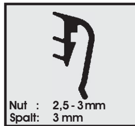
Profil-Nr. SD 2322 Farbe schwarz Material EPDM
