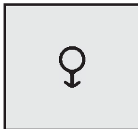
Profil-Nr. SD 2024 Farbe schwarz Material PVC
