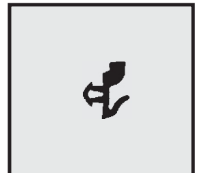
Profil-Nr. SD 2115 Farbe schwarz Material EPDM
