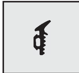
Profil-Nr. SD 2459 Farbe weiß Material Silicon
