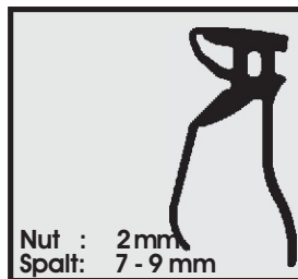
Profil-Nr. SD 2316 Farbe schwarz Material EPDM
