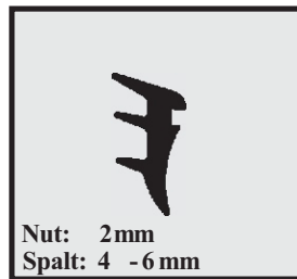
Profil-Nr. SD 2036 Farbe schwarz Material EPDM
