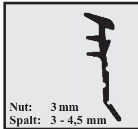
Profil-Nr. SD 2094 Farbe schwarz Material EPDM
