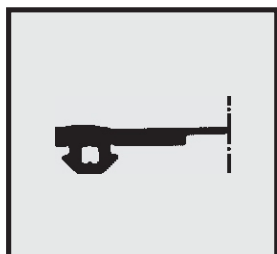
Profil-Nr. SD 2391 Farbe schwarz Material EPDM
