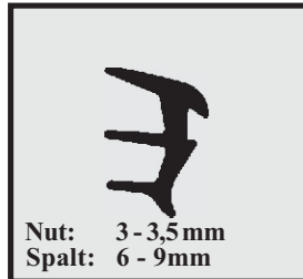
Profil-Nr. SD 2083 Farbe schwarz Material EPDM
