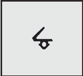
Profil-Nr. SD 2143 Farbe schwarz Material EPDM
