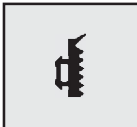
Profil-Nr. SD 2298 Farbe schwarz Material EPDM
