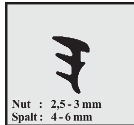
Profil-Nr. SD 2042 Farbe schwarz Material EPDM
