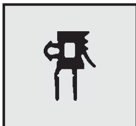
Profil-Nr. SD 2387 Farbe schwarz Material EPDM
