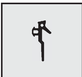
Profil-Nr. SD 2382 Farbe schwarz Material EPDM
