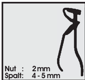
Profil-Nr. SD 2314 Farbe schwarz Material EPDM
