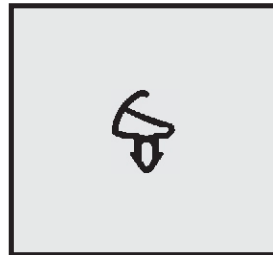
Profil-Nr. SD 2115 Farbe schwarz Material EPDM
