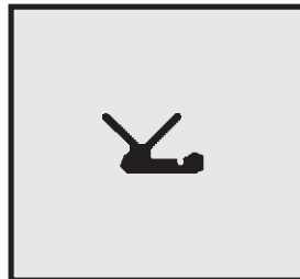
Profil-Nr. SD 2109 Farbe schwarz Material EPDM
