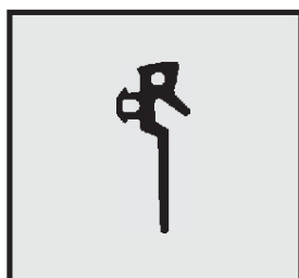
Profil-Nr. SD 22381 Farbe schwarz Material EPDM
