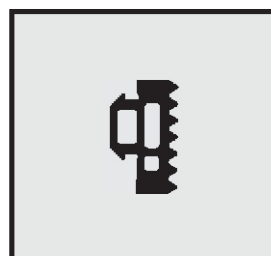
Profil-Nr. SD 2225 Farbe schwarz Material EPDM
