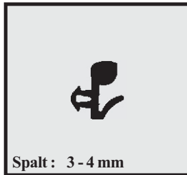
Profil-Nr. SD 2175 Farbe schwarz Material EPDM
