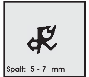
Profil-Nr. SD 2136 Farbe schwarz Material EPDM
