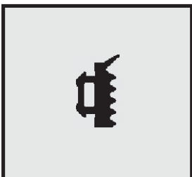
Profil-Nr. SD 2297 Farbe schwarz Material EPDM
