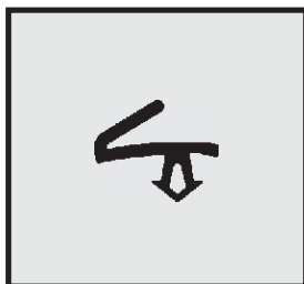
Profil-Nr. SD 2022 Farbe schwarz Material EPDM
