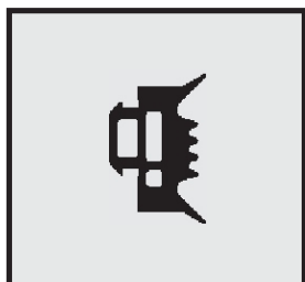
Profil-Nr. SD 2307 Farbe schwarz Material EPDM
