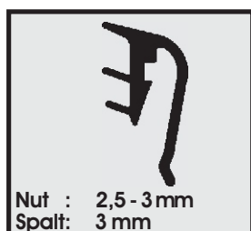
Profil-Nr. SD 2333 Farbe schwarz Material EPDM
