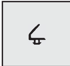
Profil-Nr. SD 2478 Farbe schwarz Material EPDM
