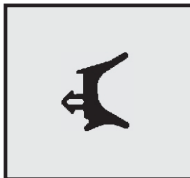
Profil-Nr. SD 2133 Farbe schwarz Material EPDM
