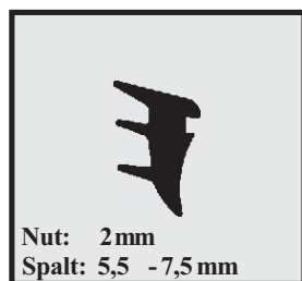
Profil-Nr. SD 2037 Farbe schwarz Material EPDM
