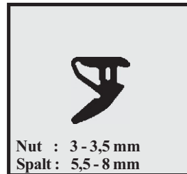
Profil-Nr. SD 2374 Farbe schwarz Material EPDM
