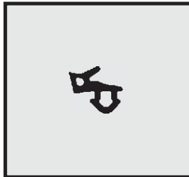
Profil-Nr. SD 2164 Farbe grau Material EPDM
