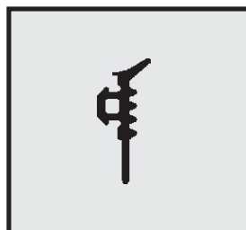
Profil-Nr. SD 2317 Farbe schwarz Material EPDM
