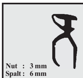
Profil-Nr. SD 2403 Farbe schwarz Material EPDM
