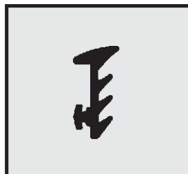
Profil-Nr. SD 2030 Farbe schwarz Material EPDM
