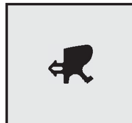
Profil-Nr. SD 2119 Farbe schwarz Material EPDM
