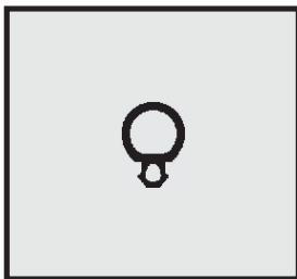
Profil-Nr. SD 2034 Farbe schwarz Material EPDM
