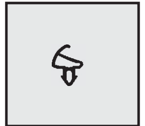
Profil-Nr. SD 2116 Farbe grau Material EPDM
