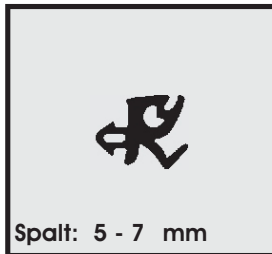
Profil-Nr. SD 2128 Farbe schwarz Material EPDM
