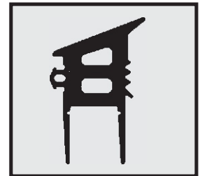
Profil-Nr. SD 2380 Farbe schwarz Material EPDM
