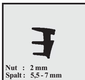
Profil-Nr. SD 2264 Farbe schwarz Material EPDM
