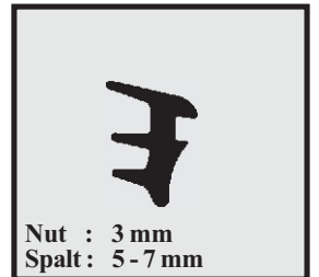
Profil-Nr. SD 2460 Farbe schwarz Material EPDM
