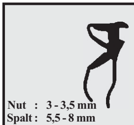
Profil-Nr. SD 2373 Farbe schwarz Material EPDM
