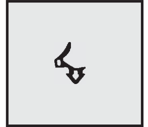
Profil-Nr. SD 2106 Farbe schwarz Material EPDM
