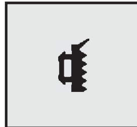
Profil-Nr. SD 2300 Farbe schwarz Material EPDM
