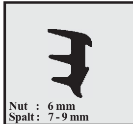
Profil-Nr. SD 2211 Farbe schwarz Material EPDM
