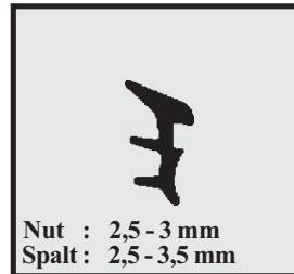
Profil-Nr. SD 2221 Farbe schwarz Material Silicon
