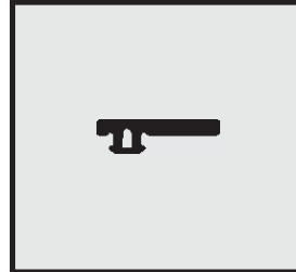
Profil-Nr. SD 2449 Farbe schwarz Material EPDM
