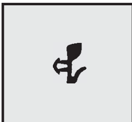
Profil-Nr. SD 2117 Farbe schwarz Material EPDM
