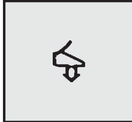
Profil-Nr. SD 2185 Farbe schwarz Material EPDM
