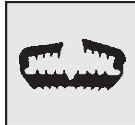
Profil-Nr. SD 2354 Farbe schwarz Material EPDM
