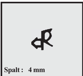
Profil-Nr. SD 2153 Farbe schwarz Material EPDM
