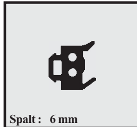
Profil-Nr. SD 2468 Farbe schwarz Material EPDM
