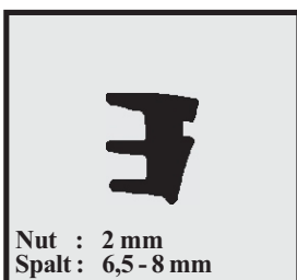
Profil-Nr. SD 2243 Farbe schwarz Material EPDM
