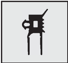
Profil-Nr. SD 2366 Farbe schwarz Material EPDM
