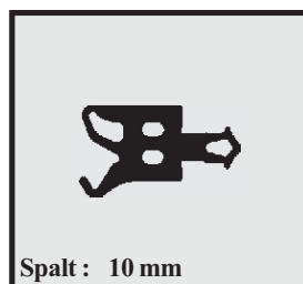
Profil-Nr. SD 2404 Farbe schwarz Material EPDM
