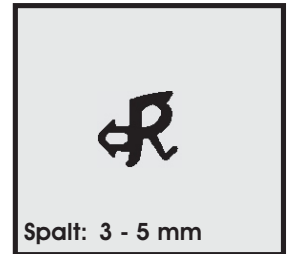
Profil-Nr. SD 2126 Farbe schwarz Material EPDM
