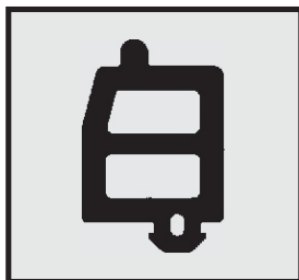
Profil-Nr. SD 2253 Farbe schwarz Material EPDM
