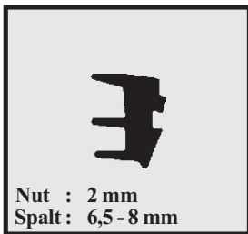
Profil-Nr. SD 2259 Farbe schwarz Material EPDM
