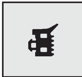
Profil-Nr. SD 2260 Farbe schwarz Material EPDM
