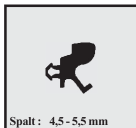
Profil-Nr. SD 2180 Farbe schwarz Material EPDM
