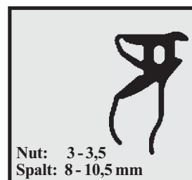
Profil-Nr. SD 2364 Farbe schwarz Material EPDM
