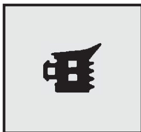
Profil-Nr. SD 2258 Farbe schwarz Material EPDM
