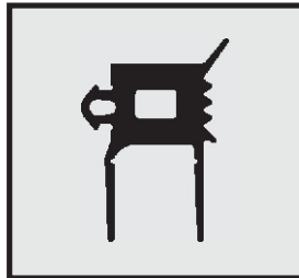
Profil-Nr. SD 2368 Farbe schwarz Material EPDM
