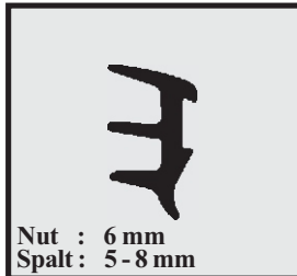
Profil-Nr. SD 2210 Farbe schwarz Material EPDM
