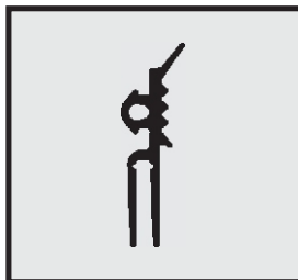
Profil-Nr. SD 2377 Farbe schwarz Material EPDM
