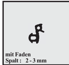
Profil-Nr. SD 2176 Farbe schwarz Material EPDM
