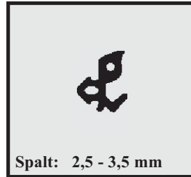
Profil-Nr. SD 2110 Farbe schwarz Material EPDM
