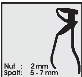
Profil-Nr. SD 2315 Farbe schwarz Material EPDM
