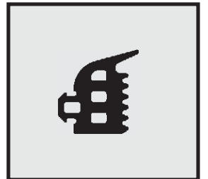
Profil-Nr. SD 2276 Farbe schwarz Material EPDM
