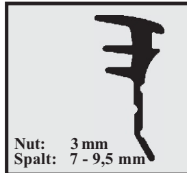
Profil-Nr. SD 2084 Farbe schwarz Material EPDM
