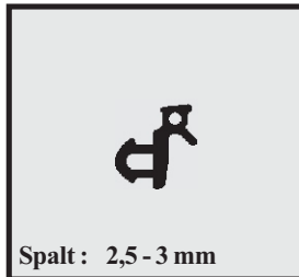
Profil-Nr. SD 2195 Farbe schwarz Material EPDM
