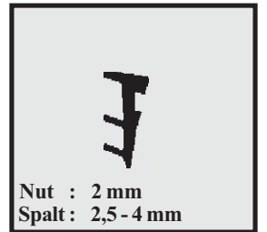
Profil-Nr. SD 2241 Farbe schwarz Material EPDM
