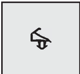
Profil-Nr. SD 2168 Farbe schwarz Material EPDM
