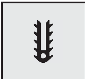
Profil-Nr. SD 2214 Farbe schwarz Material EPDM
