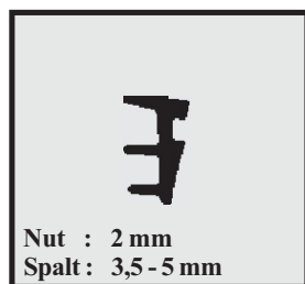
Profil-Nr. SD 2262 Farbe schwarz Material EPDM
