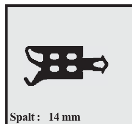
Profil-Nr. SD 2405 Farbe schwarz Material EPDM
