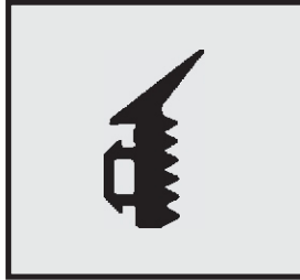
Profil-Nr. SD 2229 Farbe schwarz Material EPDM
