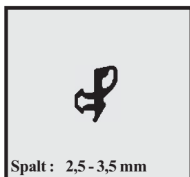
Profil-Nr. SD 2178 Farbe schwarz Material EPDM
