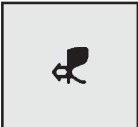
Profil-Nr. SD 2188 Farbe Pap.weiß Material EPDM
