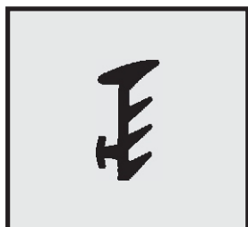
Profil-Nr. SD 2027 Farbe schwarz Material EPDM
