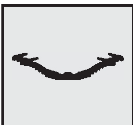
Profil-Nr. SD 2402 Farbe schwarz Material EPDM
