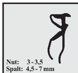
Profil-Nr. SD 2363 Farbe schwarz Material EPDM
