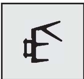
Profil-Nr. SD 2324 Farbe schwarz Material EPDM
