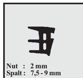
Profil-Nr. SD 2266 Farbe schwarz Material EPDM
