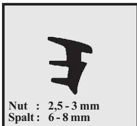
Profil-Nr. SD 2218 Farbe schwarz Material EPDM
