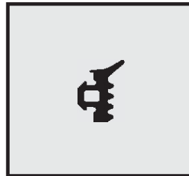
Profil-Nr. SD 2308 Farbe schwarz Material EPDM
