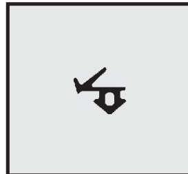
Profil-Nr. SD 2156 Farbe grau Material EPDM
