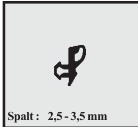
Profil-Nr. SD 2149 Farbe schwarz Material EPDM
