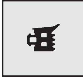
Profil-Nr. SD 2269 Farbe schwarz Material EPDM
