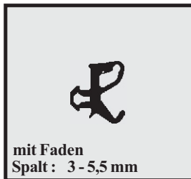
Profil-Nr. SD 2174 Farbe schwarz Material EPDM
