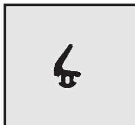
Profil-Nr. SD 2395 Farbe schwarz Material EPDM
