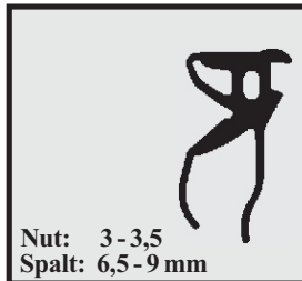
Profil-Nr. SD 2358 Farbe schwarz Material EPDM
