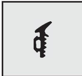
Profil-Nr. SD 2458 Farbe schwarz Material EPDM
