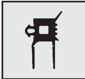
Profil-Nr. SD 2367 Farbe schwarz Material EPDM
