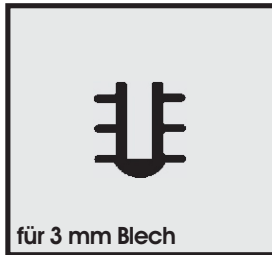
Profil-Nr. SD 2278 Farbe schwarz Material EPDM
