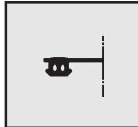
Profil-Nr. SD 2454 Farbe schwarz Material EPDM
