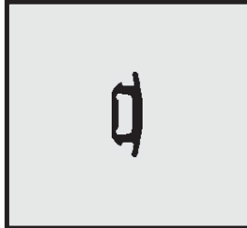
Profil-Nr. SD 2288 Farbe schwarz Material EPDM
