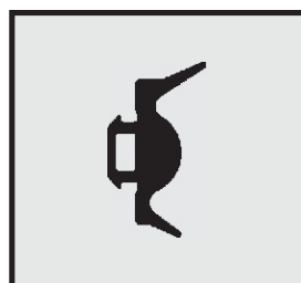
Profil-Nr. SD 2304 Farbe schwarz Material EPDM
