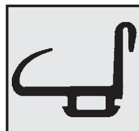
Profil-Nr. SD 2226 Farbe schwarz Material EPDM
