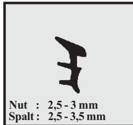
Profil-Nr. SD 2220 Farbe schwarz Material EPDM
