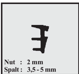
Profil-Nr. SD 2263 Farbe schwarz Material Silicon
