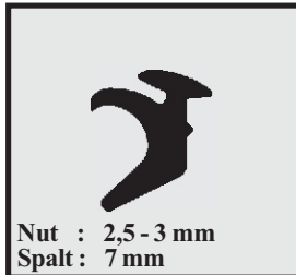
Profil-Nr. SD 2467 Farbe schwarz Material EPDM
