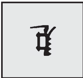
Profil-Nr. SD 2320 Farbe schwarz Material EPDM
