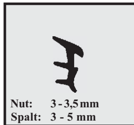
Profil-Nr. SD 2093 Farbe schwarz Material EPDM
