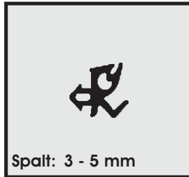
Profil-Nr. SD 2124 Farbe schwarz Material EPDM
