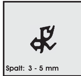
Profil-Nr. SD 2135 Farbe schwarz Material EPDM
