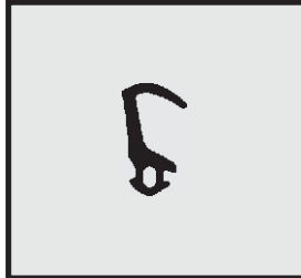
Profil-Nr. SD 2349 Farbe schwarz Material EPDM
