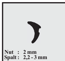
Profil-Nr. SD 2200 Farbe schwarz Material EPDM
