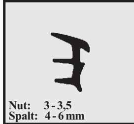
Profil-Nr. SD 2350 Farbe schwarz Material EPDM
