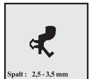
Profil-Nr. SD 2182 Farbe schwarz Material EPDM
