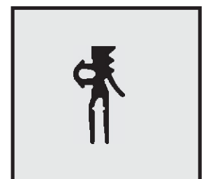
Profil-Nr. SD 2385 Farbe schwarz Material EPDM
