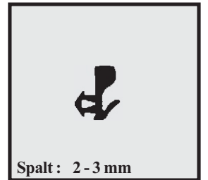
Profil-Nr. SD 2177 Farbe schwarz Material EPDM
