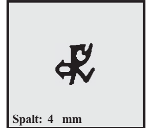
Profil-Nr. SD 2005 Farbe schwarz Material EPDM
