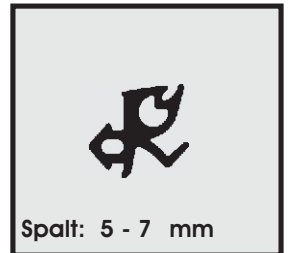
Profil-Nr. SD 2136 Farbe schwarz Material EPDM
