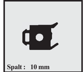
Profil-Nr. SD 2470 Farbe schwarz Material EPDM
