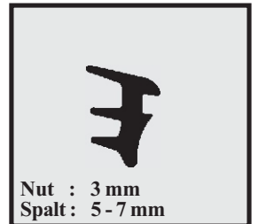
Profil-Nr. SD 2460 Farbe schwarz Material EPDM
