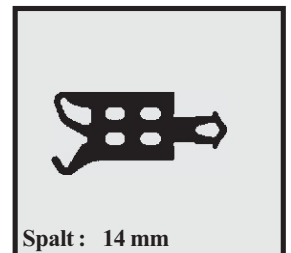
Profil-Nr. SD 2405 Farbe schwarz Material EPDM
