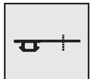
Profil-Nr. SD 2347 Farbe schwarz Material EPDM
