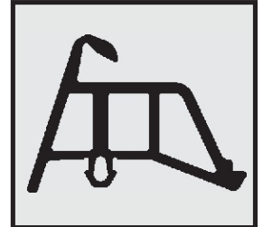
Profil-Nr. SD 2332 Farbe schwarz Material EPDM
