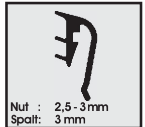
Profil-Nr. SD 2322 Farbe schwarz Material EPDM
