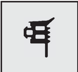
Profil-Nr. SD 2313 Farbe schwarz Material EPDM
