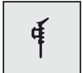
Profil-Nr. SD 2317 Farbe schwarz Material EPDM
