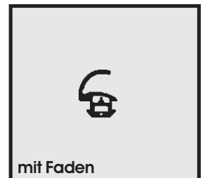
Profil-Nr. SD 2306 Farbe schwarz Material EPDM
