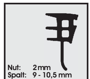
Profil-Nr. SD 2286 Farbe schwarz Material EPDM
