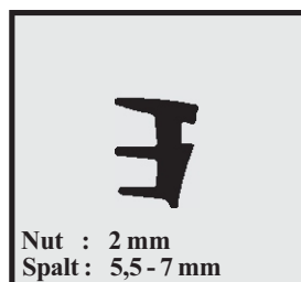
Profil-Nr. SD 2264 Farbe schwarz Material EPDM
