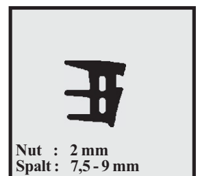
Profil-Nr. SD 2266 Farbe schwarz Material EPDM
