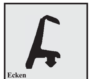
Profil-Nr. SD 2246 Farbe schwarz Material EPDM
