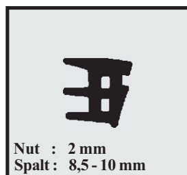
Profil-Nr. SD 2244 Farbe schwarz Material EPDM
