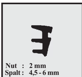
Profil-Nr. SD 2242 Farbe schwarz Material EPDM
